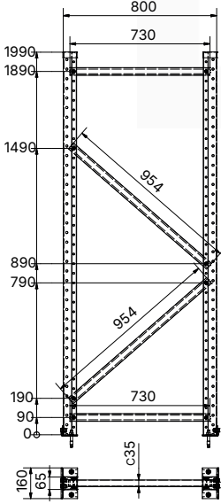
Rahmen MS 65-2,0/8 R1 Art.Nr.: RA400429
